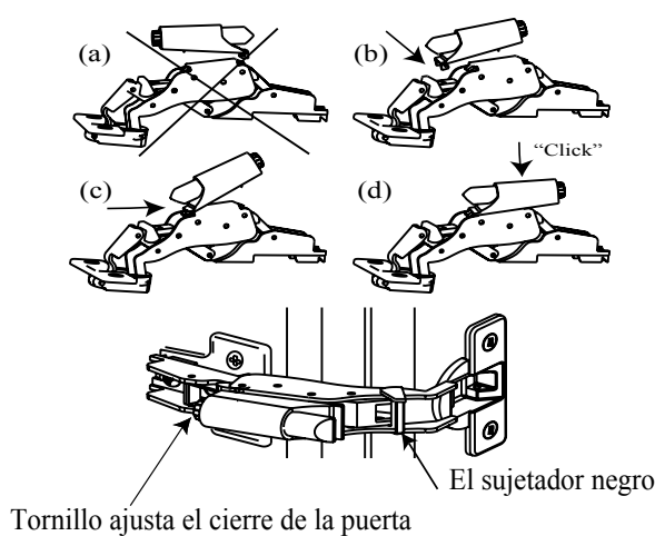
Fig. 13 Bisagra de 170 grados
